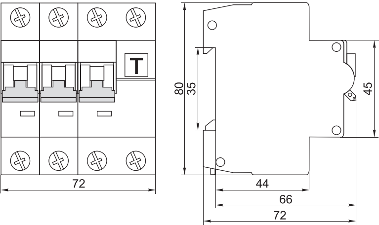
Габаритные размеры
