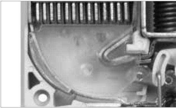
Дугоотводящая пластина подвижного контакта ВА47-60 выполнена в виде гладкой кривой, что значительно облегчает затягивание дуги в дугогасительную камеру. Помимо этого, как видно на иллюстрации, используются две пластины, что увеличивает ресурс автоматического выключателя.
