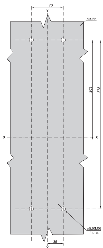
Шаблон для разметки панели
