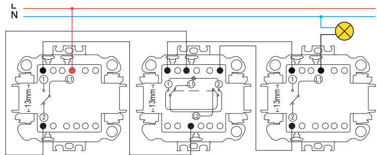
2 перемикача (з або без індикації) та 1 перехресний вимикач
