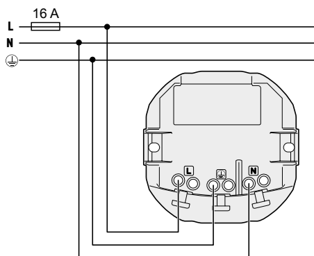
Підключення розетки 16 А
