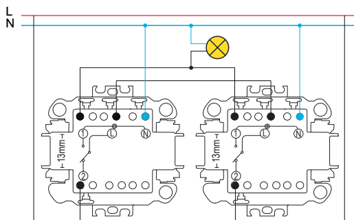
2 перемикача з індикацією
